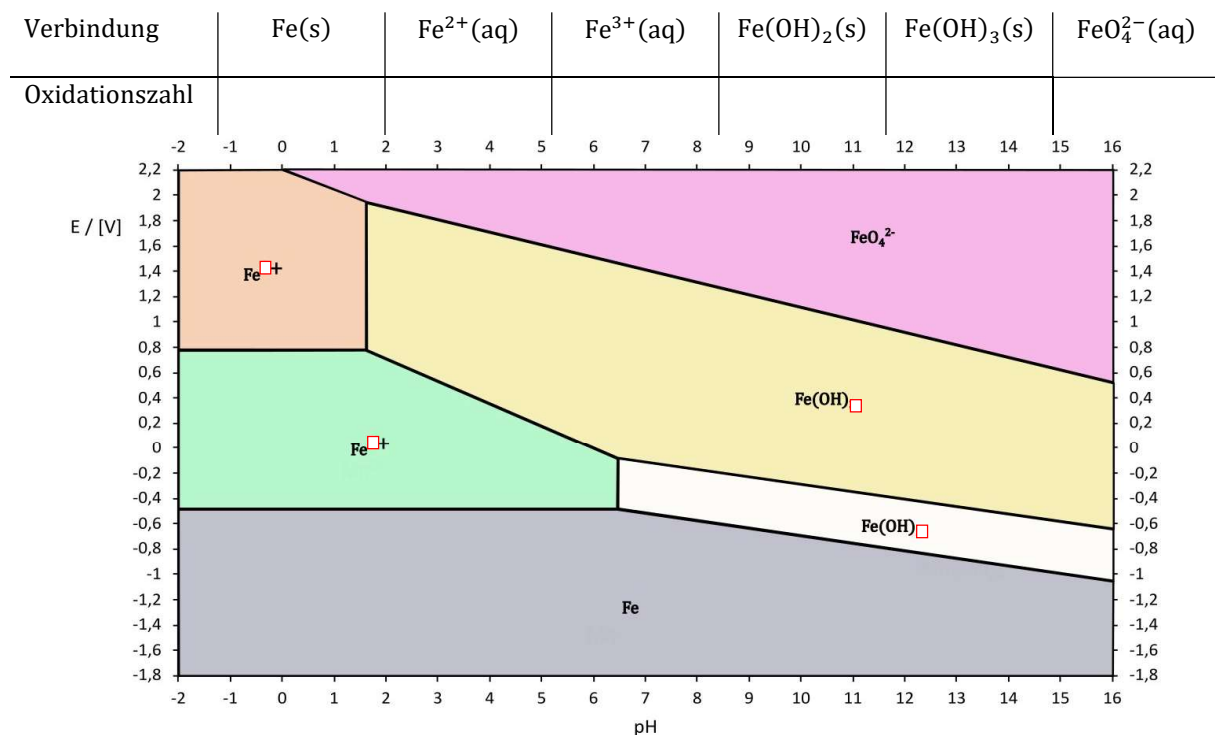
M1: Pourbaix-Diagramm für das Element Eisen bei einer Ionenkonzentration von c = 0,1 \frac{\text{mol}}{\text{L}} .
